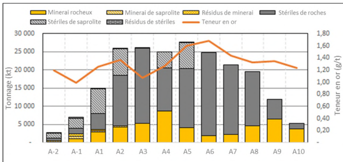
Figure 3 : Production minière annuelle
