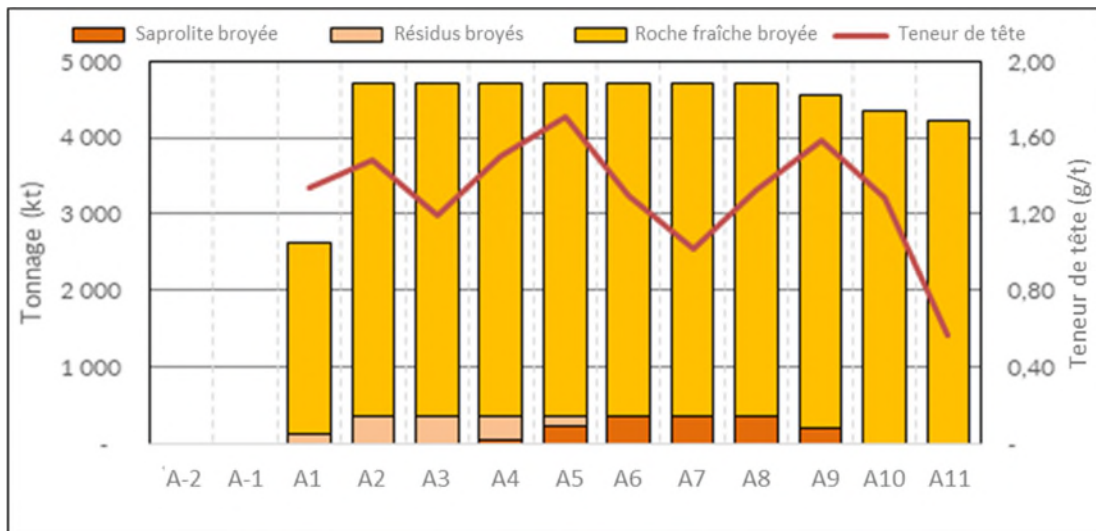
Figure 4 : Production annuelle de l'usine
